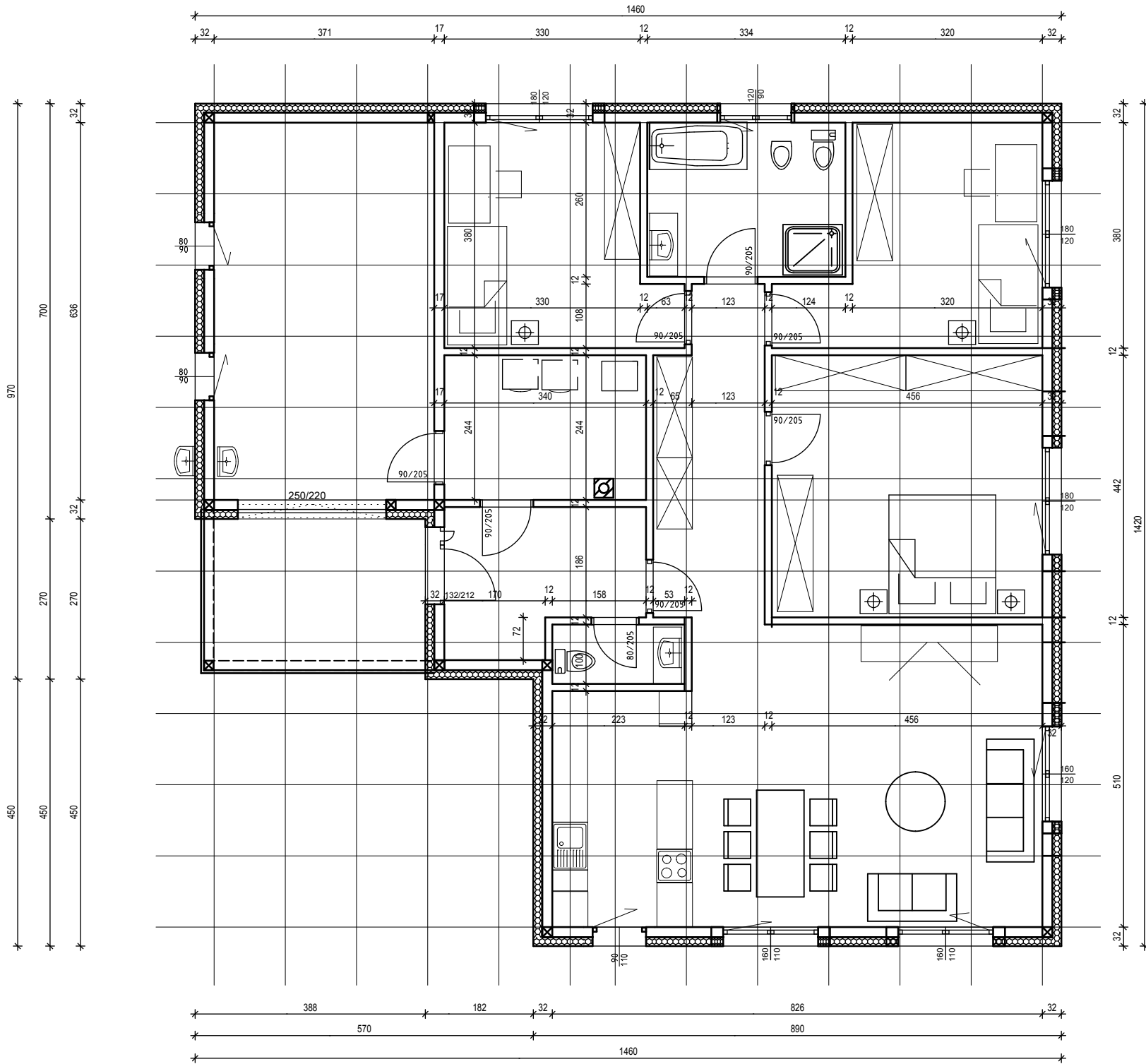
LUKS M tip 181 osnova prizemlja P=181,02m2
